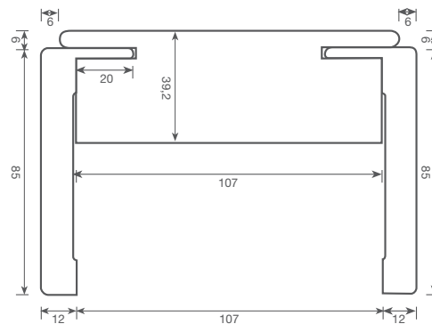
Particolare PASSATA
