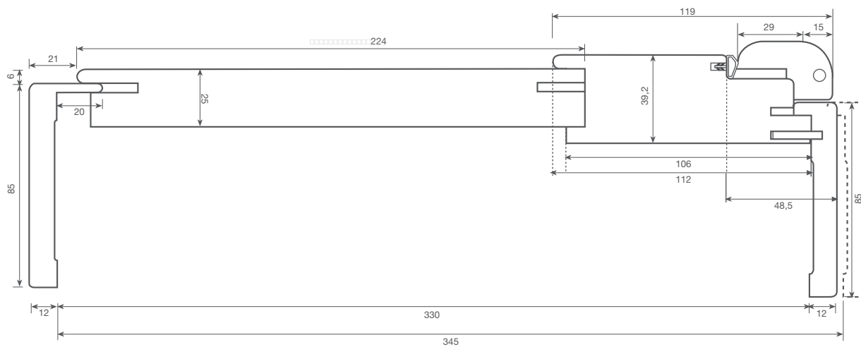
Particolare TELAIO con FOGLIO BUSSOLA
