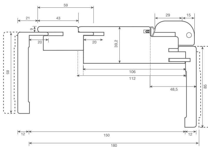
Particolare TELAIO con RINGROSSO
