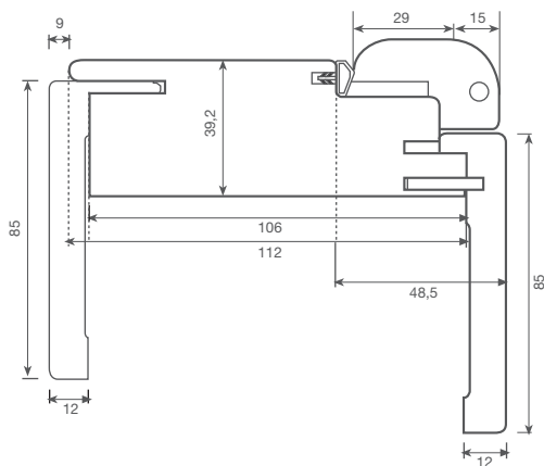
Particolare TELAIO
