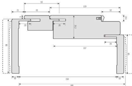
Particolare TELAIO con RINGROSSO "B"
